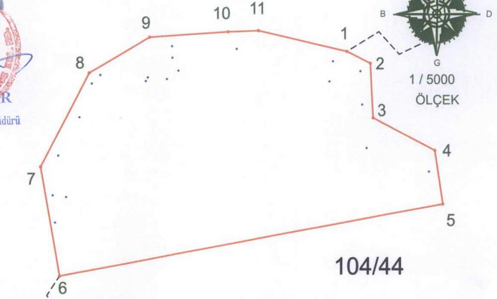
ITRF96 3 Derecelik Koordinatlar
