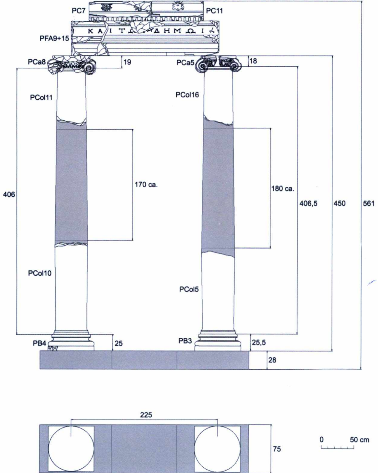
Resim 24: Sütun tamburlarının yerine yerleştirilmesi; mermer ve epoksi reçineyle tamamlanan kısımlar gri ile belirtildi.
