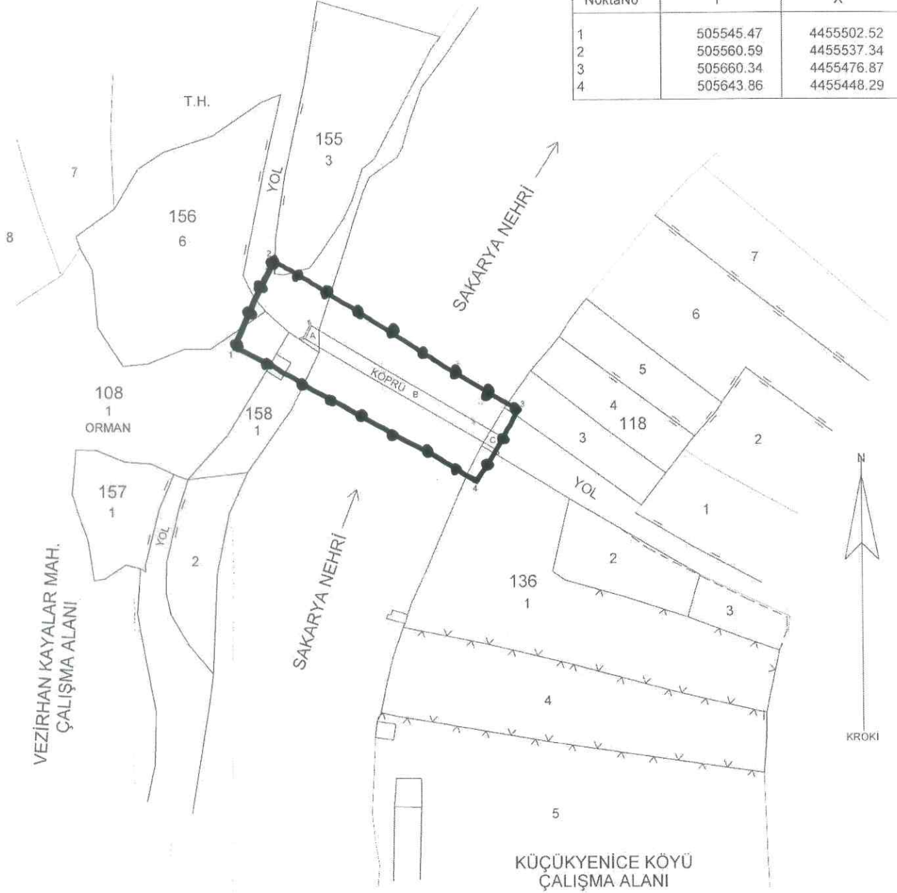
KOORDİNAT LİSTESİ ITRF_(96)
